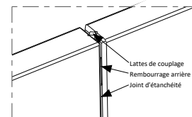
Connexion des éléments
