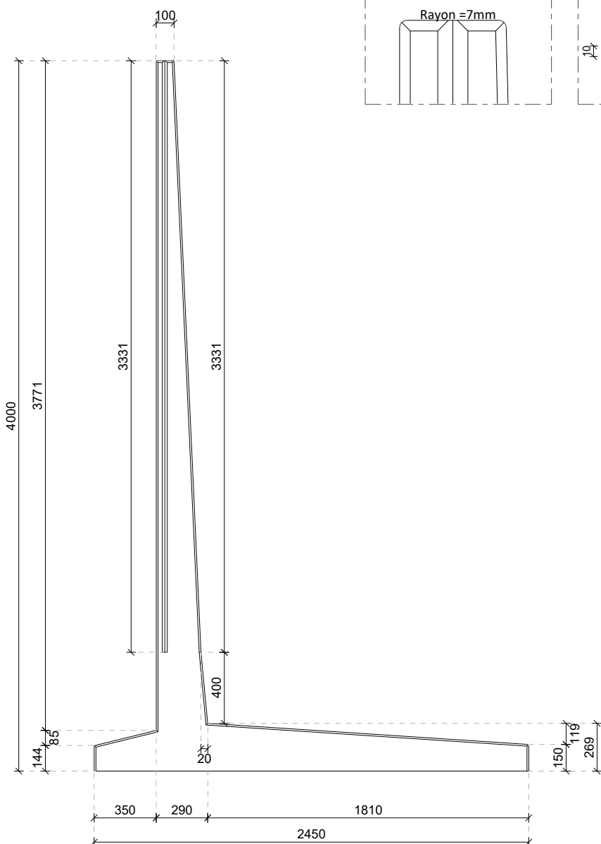
Rainure en V
